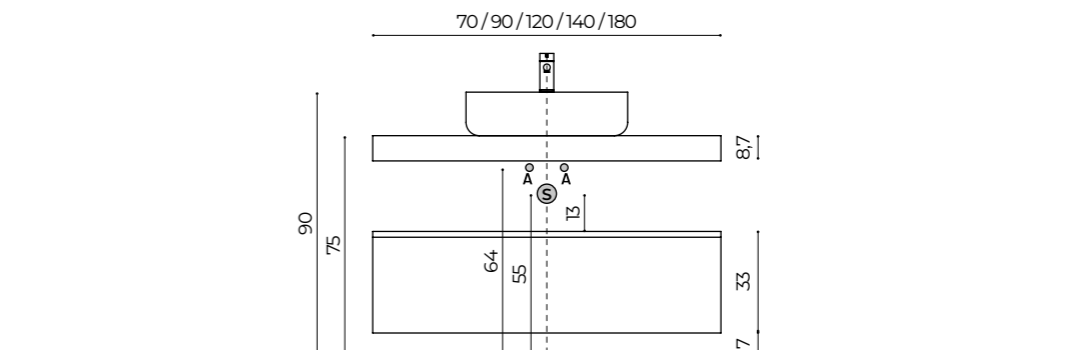
QUOTE PER TOP SCATOLARI CON BASI H.33 QUOTAS DISCHARGES FOR BOX-SHAPED TOP WITH BASE UNIT H.33
